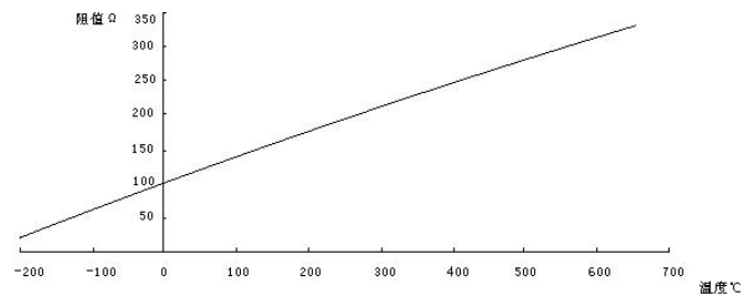
温度/电阻曲线图
