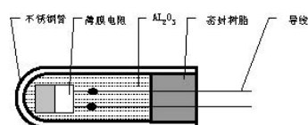
二线制电阻
