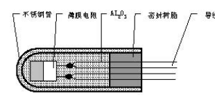
四线制电阻
