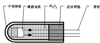
三线制电阻
