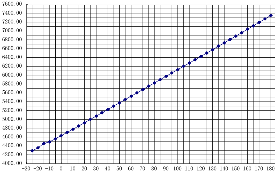
温度—阻值曲线图
