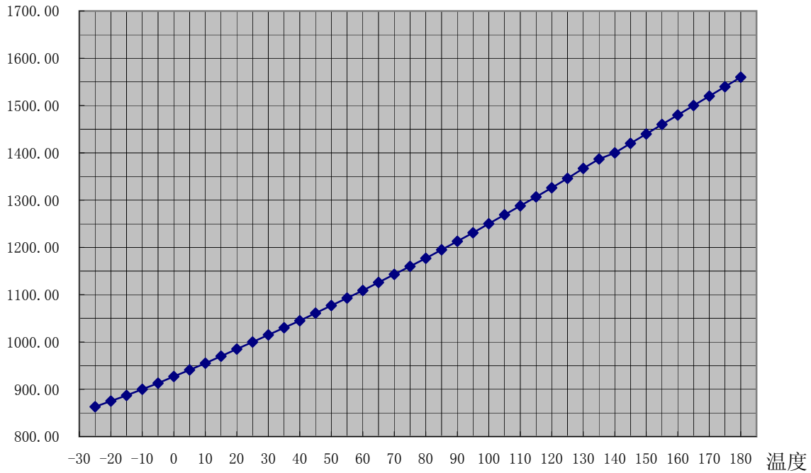
温度—阻值曲线图
